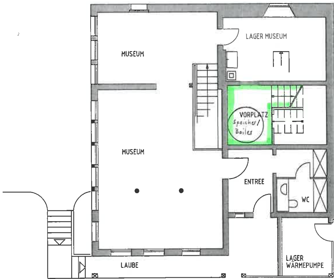
ERDGESCHOSS
